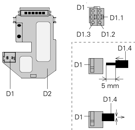
Bild 2: Anschlüsse
