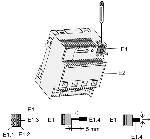
Bild 4: Busleitung anschliessen und abklemmen
