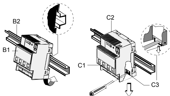
Bild 2: Montage und Demontage des Reiheneinbaugerätes
