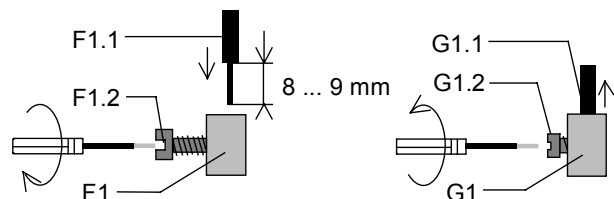
Bild 5: Laststromkreise anschliessen und abklemmen
