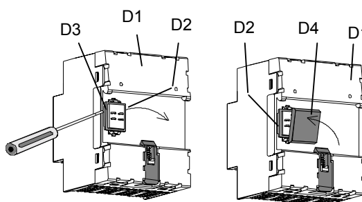
Bild 4: Abdecken des Kontaktsystems
