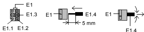
Bild 4: Busleitung anschließen und abklemmen
