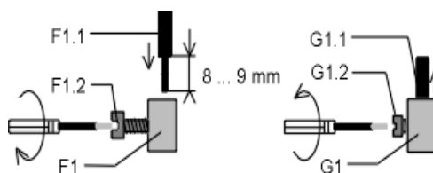
Bild 4: Laststromkreise anschließen und abklemmen
