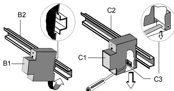
Bild 2: Montage und Demontage des Reiheneinbaugerätes
