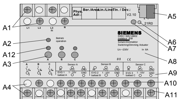
Bild 1: Lage der Anzeige- und Bedienelemente
