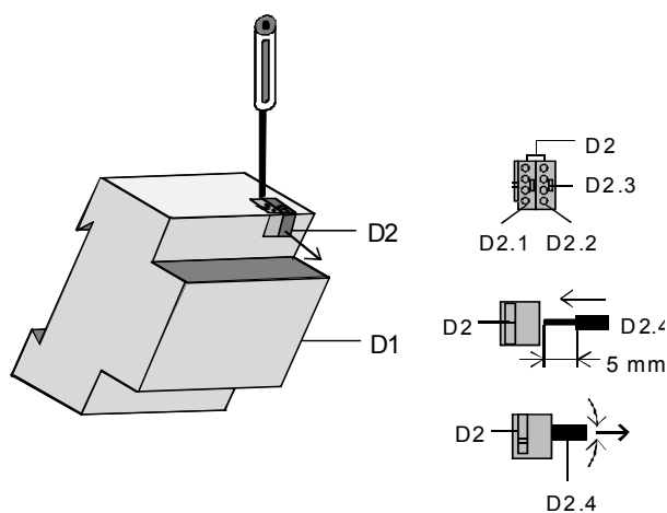
Bild 3: Busleitung anschließen und abklemmen
