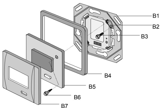
Bild 2: Montage der Anzeigeeinheit
