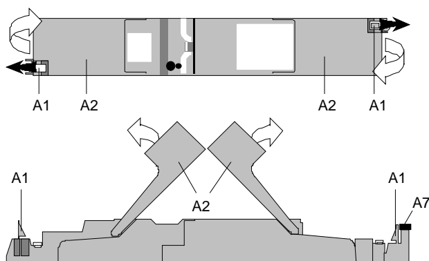
Bild 2: Öffnen und Schließen der Abdeckklappen
