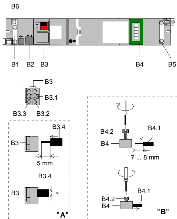
Bild 3: Anschlüsse
