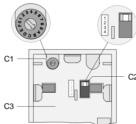
Bild 3: Einstellen des Sendekanals
