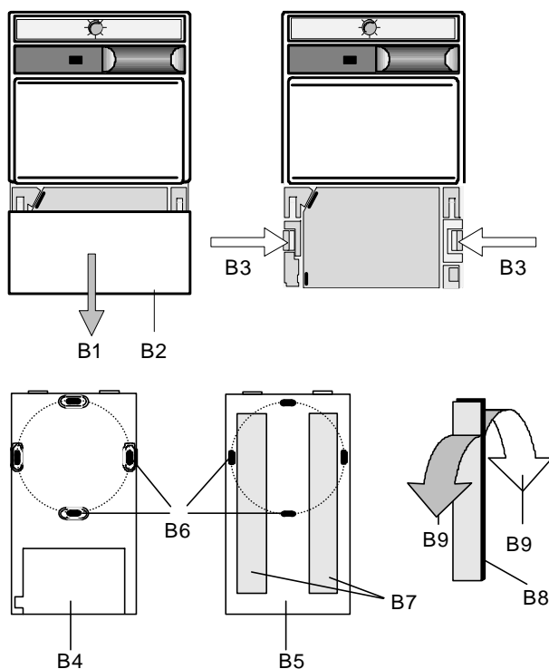
Bild 2: Montage des Wandsenders
