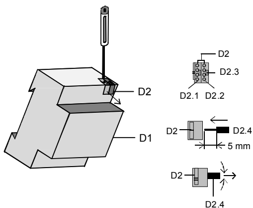
Bild 3: Busklemme aufstecken / entfernen
