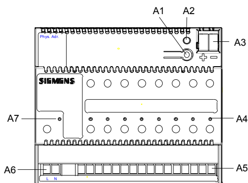
Bild 1: Lage der Anzeige- und Bedienelemente
