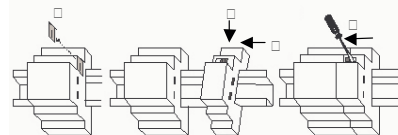
Bild 2: Wandmontage des CM EIB/KNX
