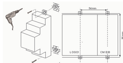
Bild 2: Wandmontage des CM EIB/KNX
