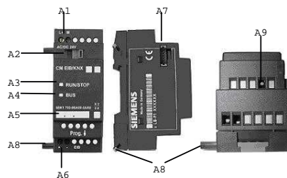
Bild 1: Lage der Anschluss- und Bedienelemente
