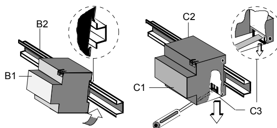
Bild 2: Montage / Demontage des Reiheneinbaugerätes
