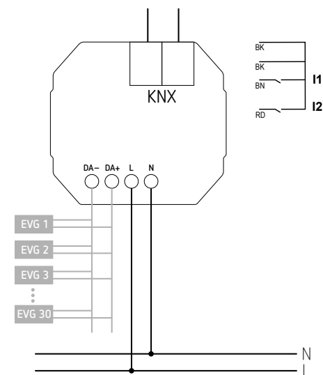
LUXORliving D1 DALI
