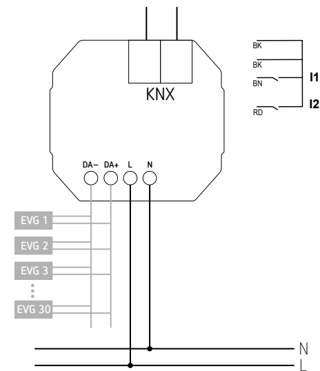
DU 1 DALI KNX
