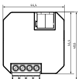
LUXORliving D1 DALI
