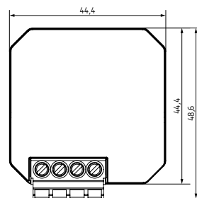
DU 1 DALI S RF KNX
