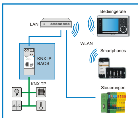
Bild 2: Typische Anwendung
