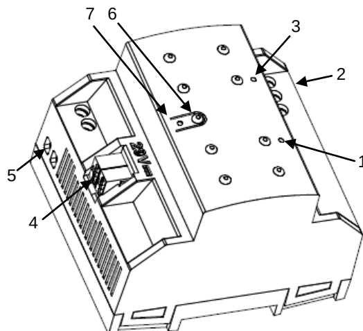
Abb. 1: ZPS320MPA230 Spannungsversorgung
