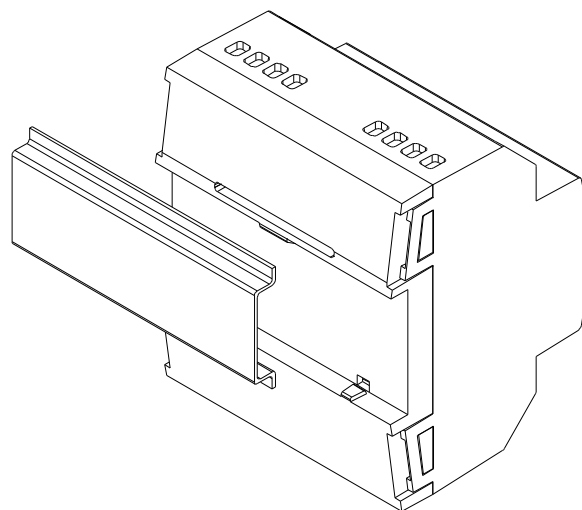
Abb. 3. MAXinBOX FANCOIL 2CH2P Hutschiennenmontage
