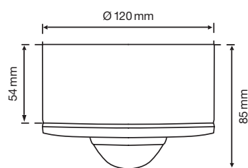
AP 360 Gehäuse IP55
