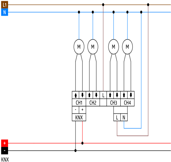
Wiring diagramms
