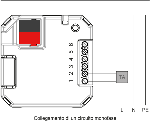
Collegamento di un circuito monofase
