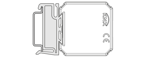
c) Ad aggancio avvenuto, collegare la linea bus e i trasformatori di corrente
