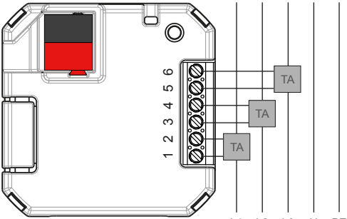
Collegamento di un circuito trifase
