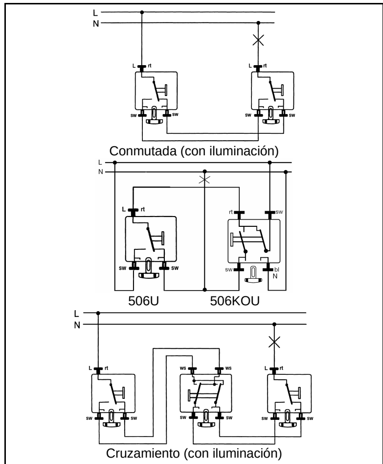
Ejemplos de conexionado 506 U
