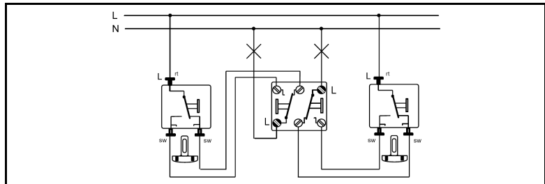
Wiring diagrams
