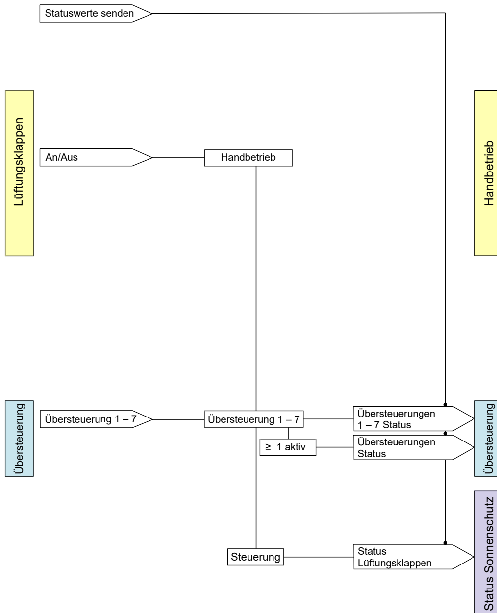
Abb. 8: Lüftungsklappen
