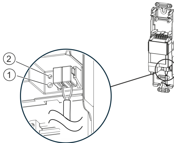
Abb. 3: Programmier Taste und Programmier-LED (Abbildung beispielhaft)
