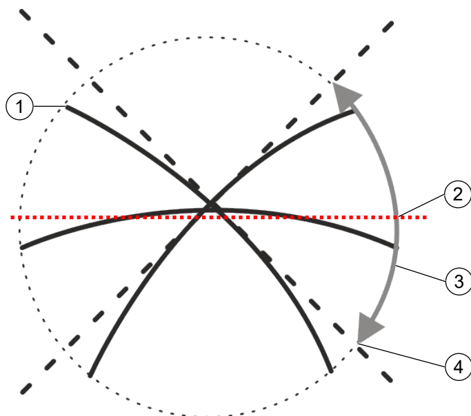
Abb. 6: Lamellenstellung im Kompatibilitätsmodus (Parametereinstellung „freigeben“)
