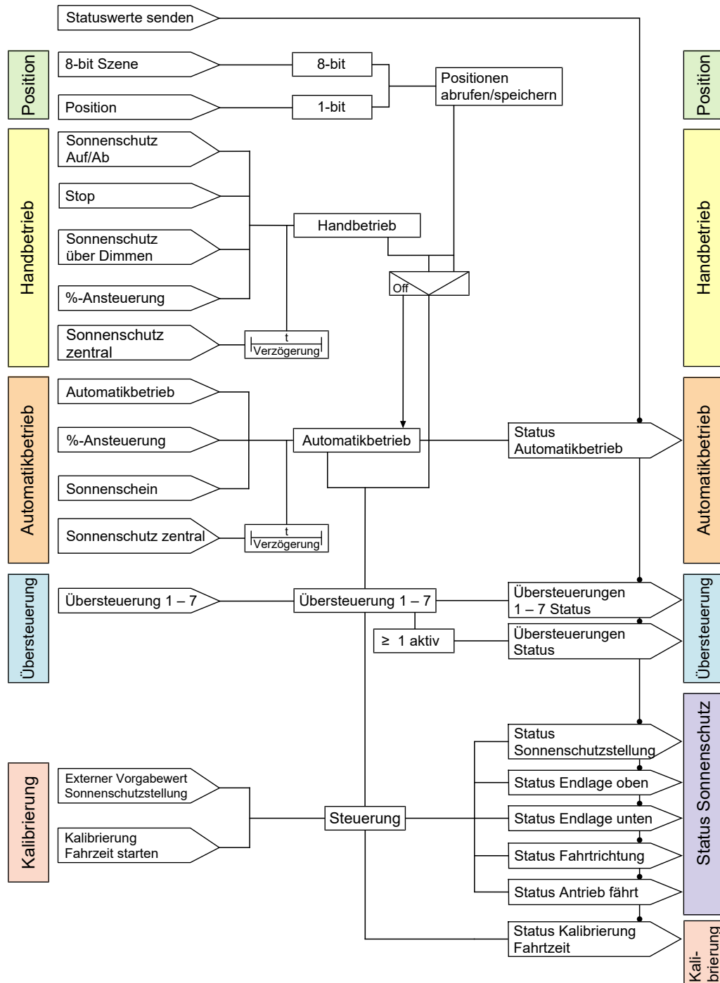
Abb. 7: Ablaufdiagramm Rollladen, Markise
