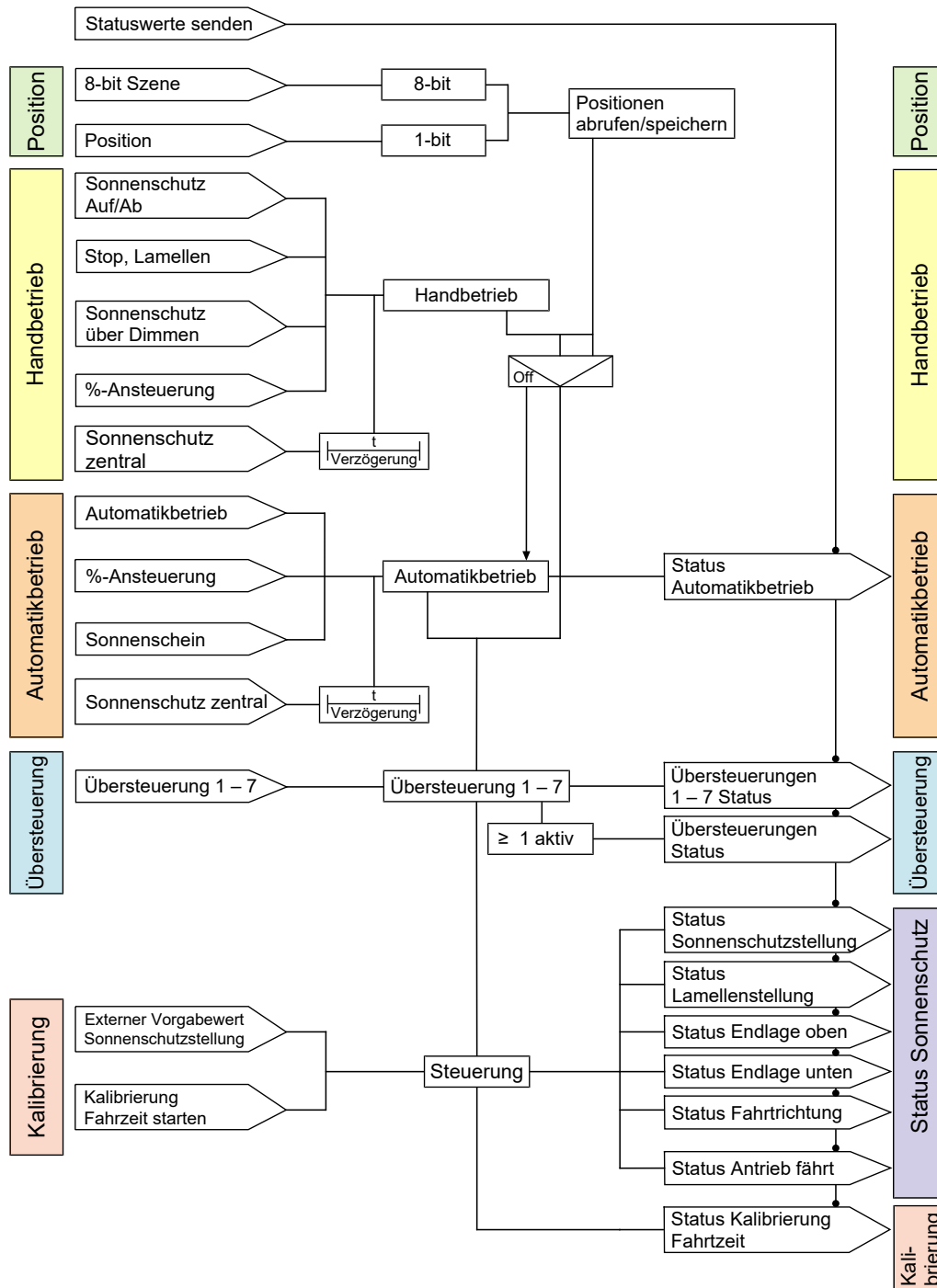
Abb. 4: Ablaufdiagramm Jalousie
