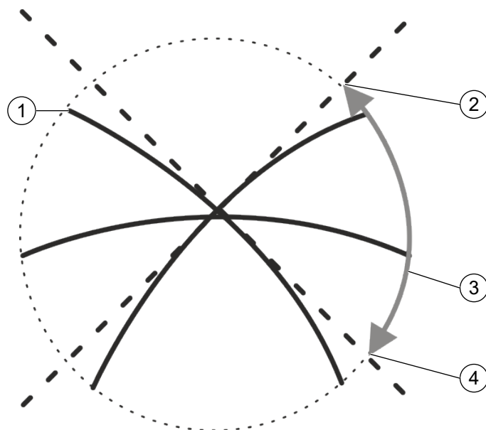
Abb. 5: Lamellenstellung nach KNX (Parametereinstellung „sperren“)
