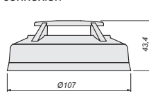
Montaje con zócalo bajo Low base assembly Montage socle bas A30XHS / A30XV / A30XT
