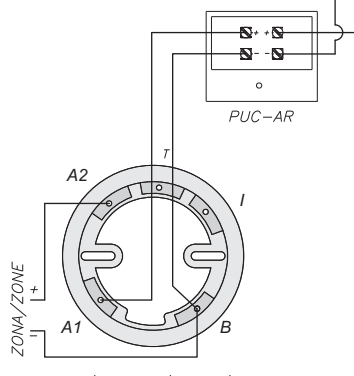
Montaje con zócalo alto High base assembly Montage socle haut A30XHS / A30XV / A30XT
