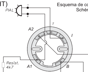
Montaje con zócalo bajo Low base assembly Montage socle bas A30XHS / A30XV / A30XT
