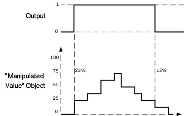
Fig12. Manipulated Value (1 Byte)
