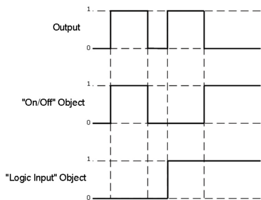
Fig10. XOR Logic Function
