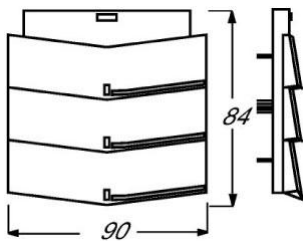
Elemento de control triton® 6320/30-500
