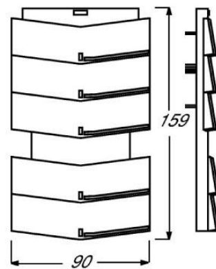
Elemento de control triton® 6320/50-500 y 6320/58-500
