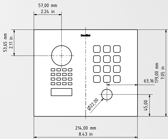
Placa frontal
