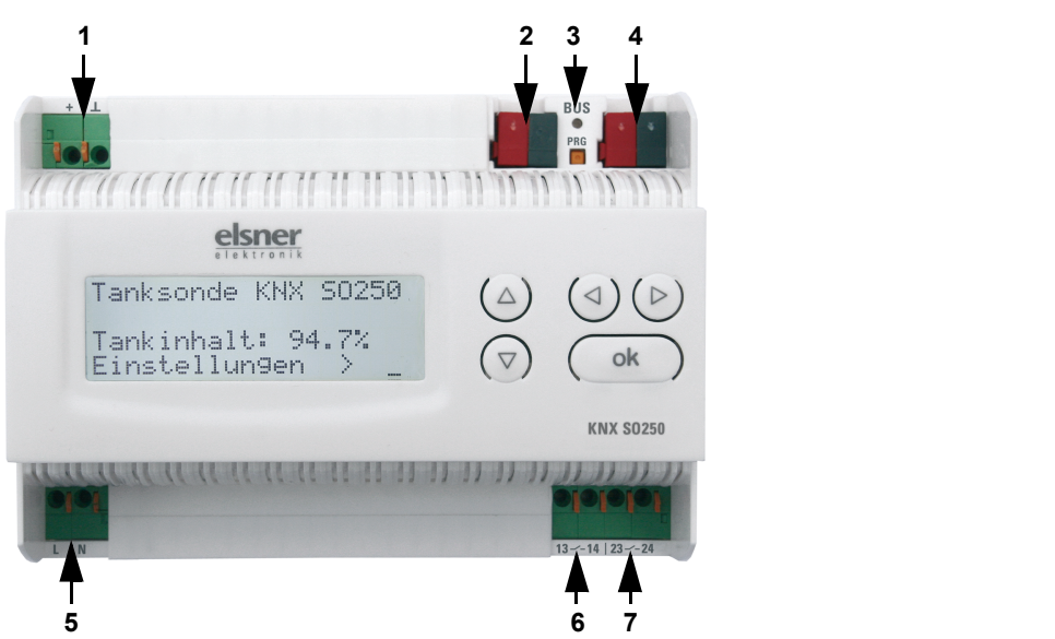
Fig. 3 1 conexión sonda de medición, + / aislamiento 2 Terminal KNX +/- 3 LED y tecla de programación 4 Terminal KNX +/- 5 entrada tensión de servicio 230 V AC, L / N 6 relé de salida 1 (contacto de cierre), 13 / 14 7 relé de salida 2 (contacto de cierre), 23 / 24 Las conexiones 1, 5, 6 y 7 son aptas para conductores sólidos de hasta 1,5 mm² o para conductores de cables finos
