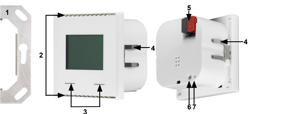
Fig. 2 1 Placa de base 2 Orificios para la circulación del aire 3 Botones táctiles 4 Pestañas 5 Terminal KNX BUS +/- 6 Tecla de programación (hundida) para programar el dispositivo 7 LED de programación (hundido)
