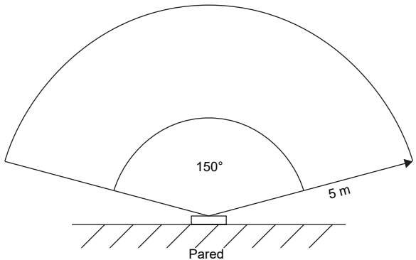
Fig. 1 horizontal (vista superior)
