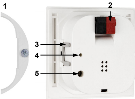
Fig. 4 Lado posterior 1 Soporte de montaje 2 Borne KNX BUS +/- 3 Encastre 4 LED de programación (hundido) 5 Tecla de programación (hundido) para programación del dispositivo
