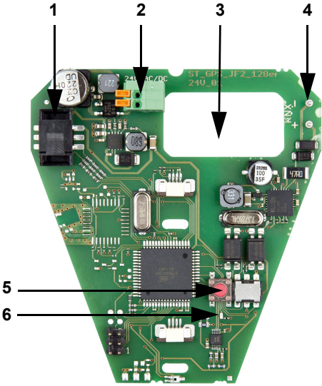
Fig. 14 1 Conexión por cable al sensor de precipitación en la tapa de la caja 2 Clema de conexión rápida para la fuente de alimentación (20...32 V DC), Cable rígido de hasta 1,5 mm² o flexible. Ocupación de bornes independiente de la polaridad (+/- o -/+) 3 Apertura para el cable de la fuente de alimentación, el cable de Bus 4 Conexión por clema de Bus KNX +/- 5 Botón de programación 6 LED de programación
