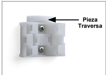
Fig. 4 Montaje en pared: lado plano hacia la pared, la pieza travesera semicircular hacia arriba.
