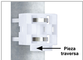
Fig. 5 Montaje en mástil: lado curvo hacia el mástil, la pieza travesera hacia abajo.
