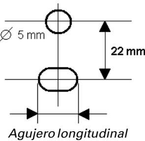
Fig. 8 a+b Esquema de taladrado
