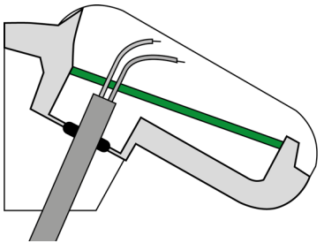
Fig. 10 Coloque el revestimiento del cable por debajo de la placa de circuitos impresos y conduzca solo los cables de conexión por las aberturas en la placa hacia arriba.
