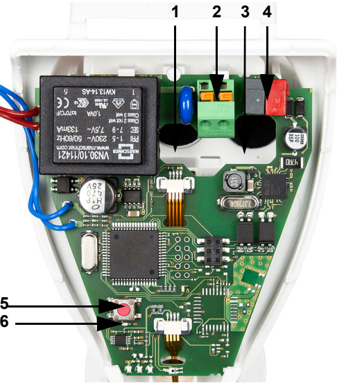
Fig. 11 1 Apertura para el cable de la fuente de alimentación 2 Clema de conexión rápida para la fuente de alimentación (230 V AC), apropiada para cable rígido de hasta 1,5 mm 2 o flexible. 3 Apertura para el cable de Bus 4 Clema de Bus KNX +/- 5 Botón de programación 6 LED de programación
