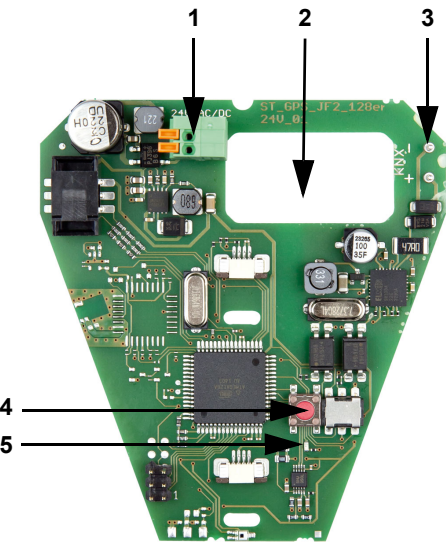
Fig. 12 1 Clema de conexión rápida para la fuente de alimentación (20...32 V DC), Cable rígido de hasta 1,5 mm 2 o flexible. Ocupación de bornes independiente de la polaridad (+/- o -/+) 2 Apertura para el cable de la fuente de alimentación, el cable de Bus 3 Conexión por clema de Bus KNX +/- 4 Botón de programación 5 LED de programación
