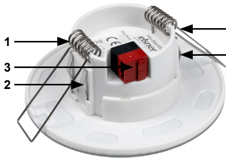
Fig. 1 1 Bornes para la instalación en techo hueco 2 Resortes para la instalación en el anillo de soporte 3 Bornes KNX
