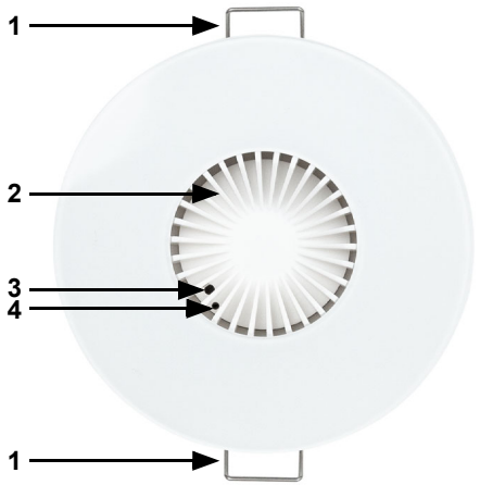
Fig. 2 1 Bornes para la instalación en techo hueco 2 Láminas de ventilación 3 Pulsador de programación (hundido, abertura de mayor tamaño) 4 LED de programación (hundido, abertura de menor tamaño)
