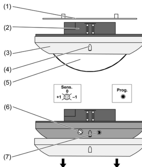
Imagen 1: Estructura del mecanismo
