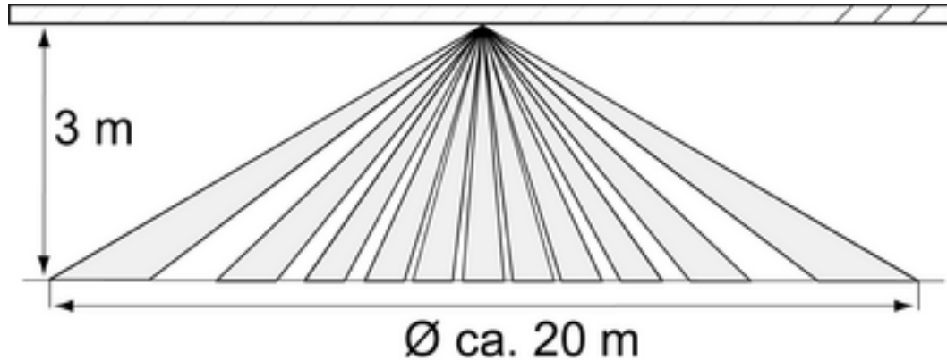
Imagen 2: Ventana del sensor y área de detección
