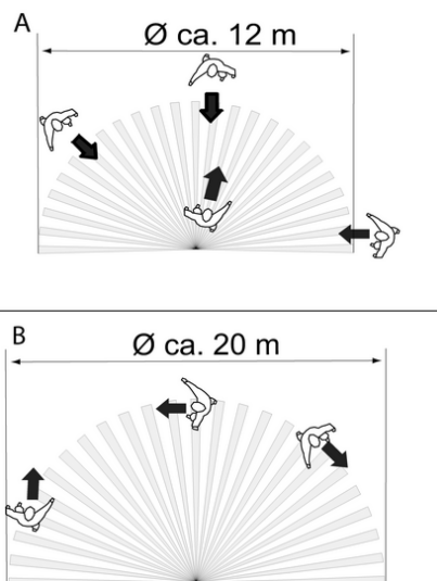
Imagen 3: El alcance de la detección depende de la dirección del movimiento con una altura de montaje de 3 m
