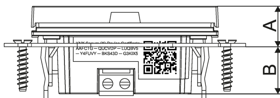
Imagen 11: Dimensiones de montaje
