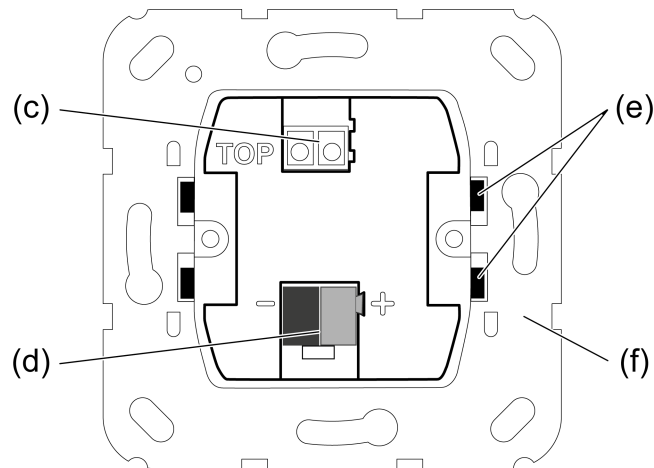
Imagen 3: Parte trasera de la estructura del aparato
