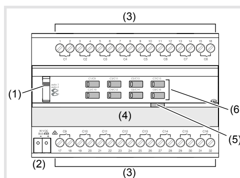
Figura 1: Ejemplo de dispositivo de 16/8 elementos
