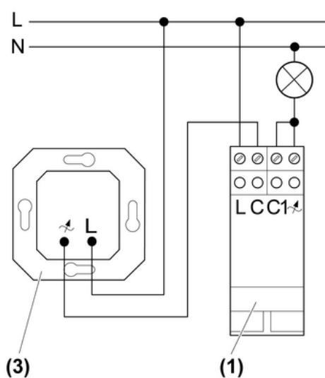
Figura 3: Plano de conexión con regulador de luz empotrado UP
