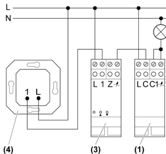
Figura 2: Plano de conexión con regulador de luz REG
