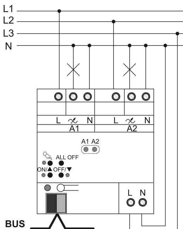
Imagen 4: Actuador de regulación – Ejemplo de conexión
