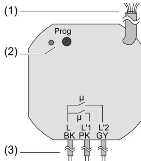
Figura 2: Actuador de conmutación doble
