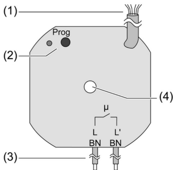
Figura 1: Actuador de conmutación simple
