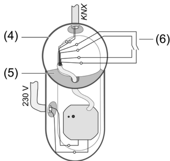
Figura 3: Montaje en caja para mecanismos
