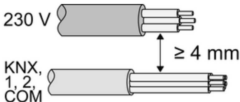
Figura 4: Distancia entre línea de red y línea piloto
