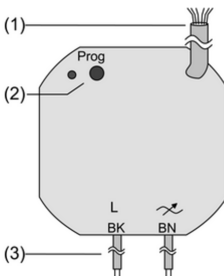
Figura 1: Actuador de regulación empotrable
