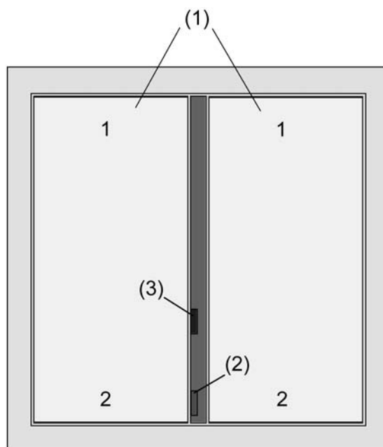
Imagen 1: Esquema del módulo sensor TSM estándar de 1 fase
