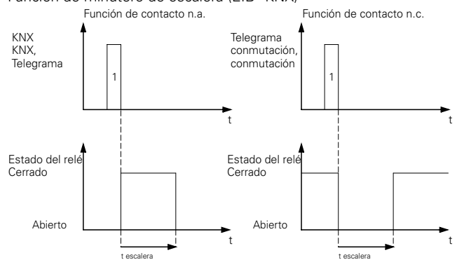
Función de minuterero de escalera (EIB=KNX)
