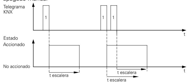
Función de minuterero de escalera no redisparable sin función de apagado manual
