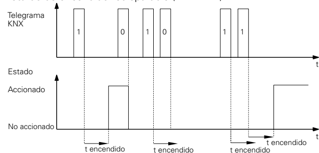
Retardo de encendido redisparable (EIB=KNX)
