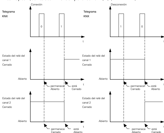
Interruptor (contacto inversor para canal 1/2) (EIB=KNX)
