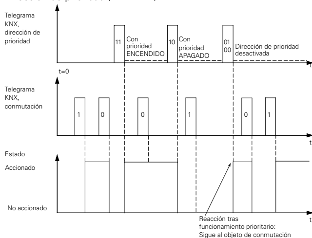
Dirección de prioridad (EIB=KNX)
