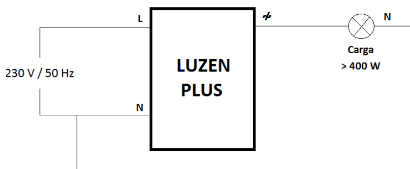
Figura 2.15. Sobrecarga
