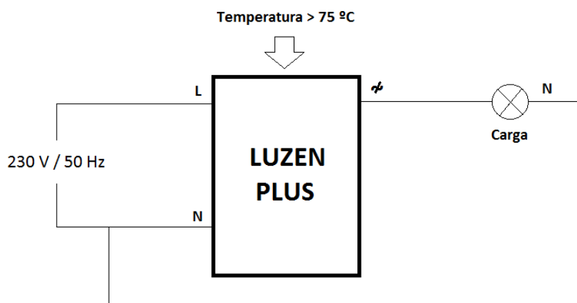
Figura 2.16. Sobretemperatura
