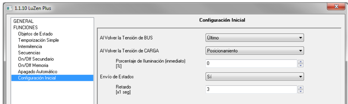
Figura 2.11. Configuración inicial
