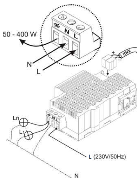
Figura 1.2. Esquema conexionado LUZEN PLUS
