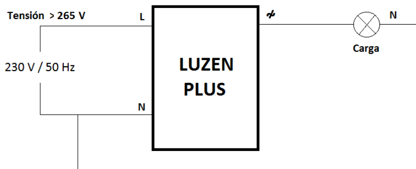
Figura 2.17. Sobretensión
