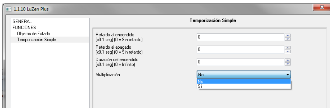
Figura 2.5. Función de Temporización Simple
