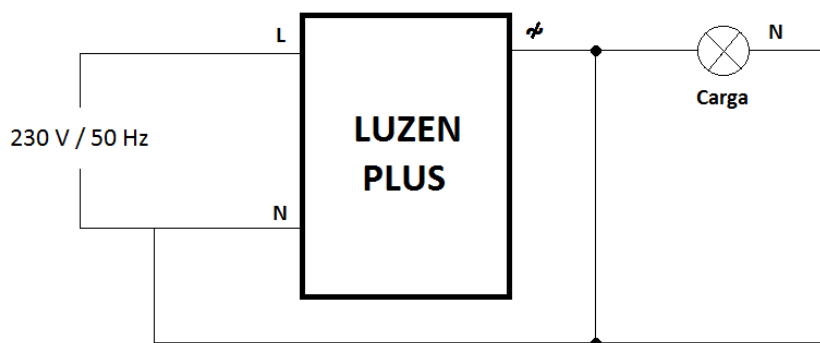
Figura 2.14. Cortocircuito
