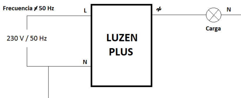
Figura 2.18. Frecuencia anómala
