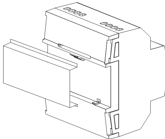
Figura 3. Anclaje en carril DIN
