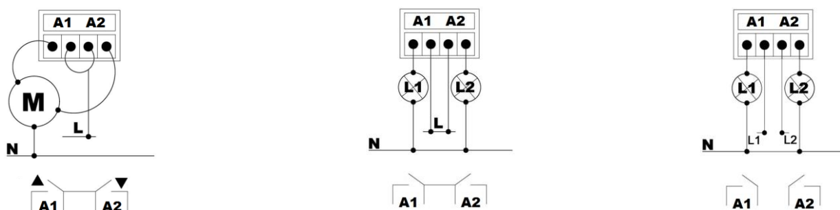
Figura 2. Ejemplos de conexiones Bloque 1 canal persiana, salidas con misma fase y salidas con fases diferentes
