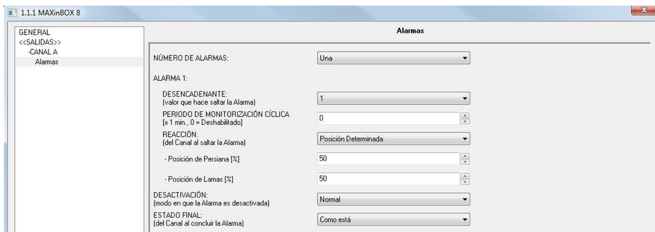
Figura 3.15. Pantalla de alarmas
