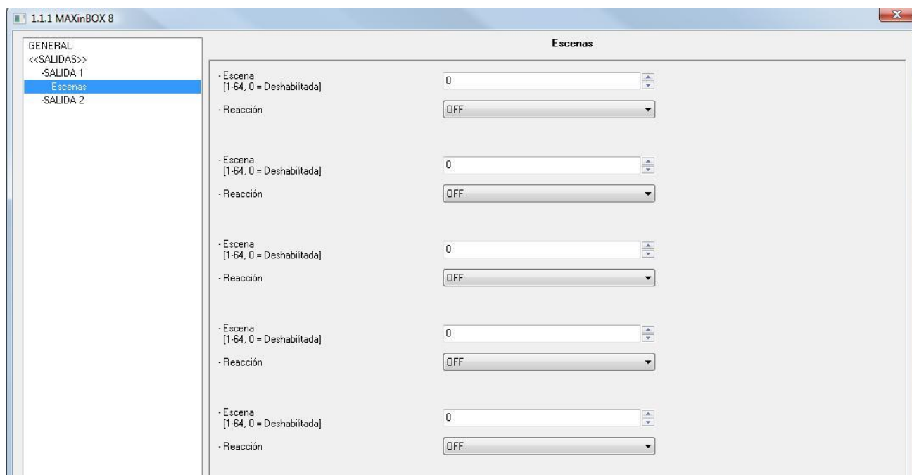
Figura 3.8. Pantalla de escenas
