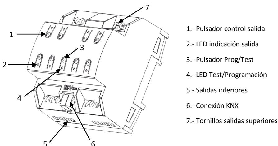
Figura 1.2. MAXinBOX 8. Esquema de elementos
