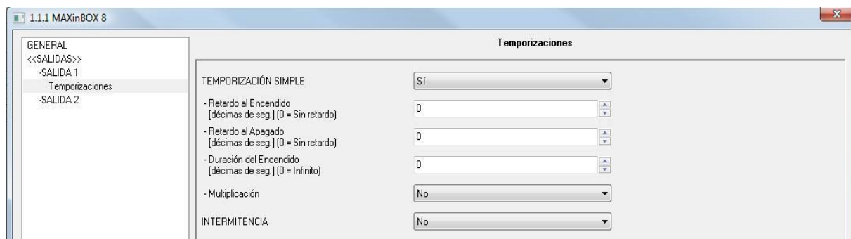
Figura 3.6. Pantalla de temporizaciones. Temporización simple
