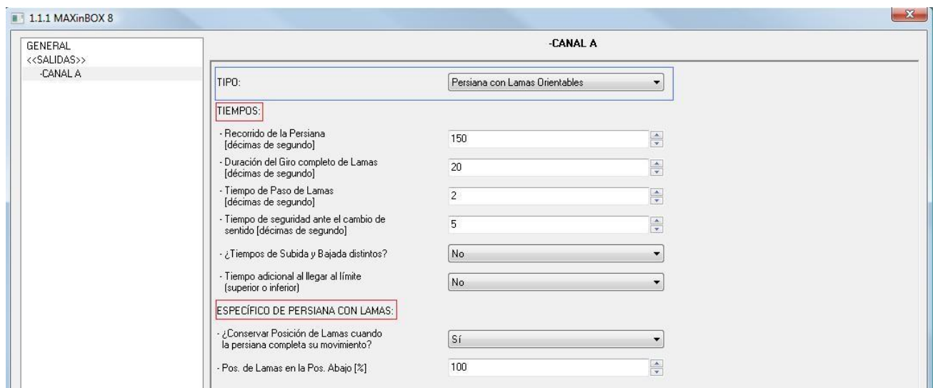
Figura 4.2. Pantalla configuración de persiana con lamas en ETS
