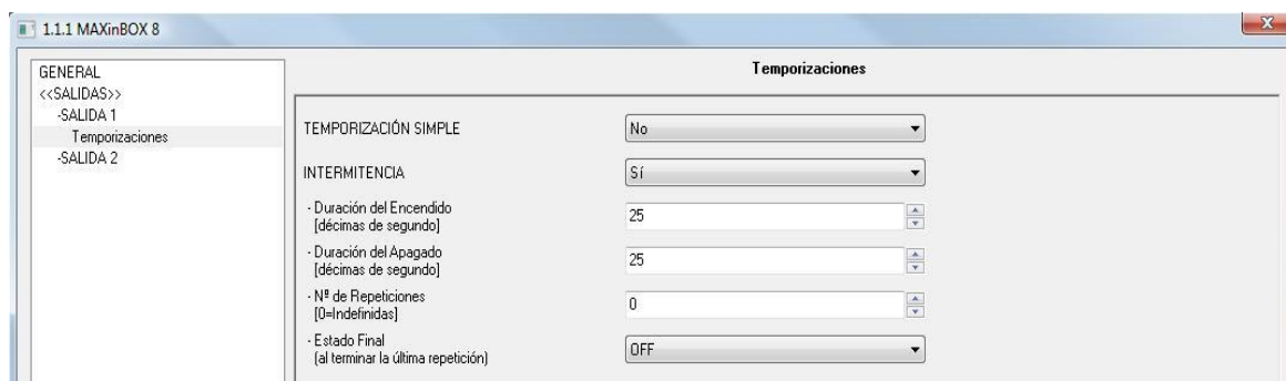
Figura 3.7. Pantalla de temporizaciones. Intermitencia.
