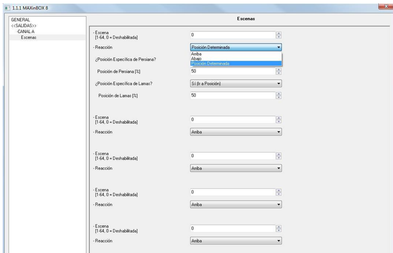
Figura 3.14. Pantalla de escenas
