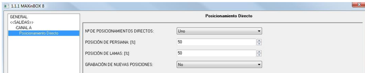
Figura 3.17. Pantalla de Posicionamiento Directo
