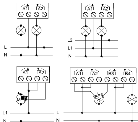
Figura 2: Ejemplo de conexionado (de izquierda a derecha y arriba a abajo): 2 cargas, 2 cargas a fases distintas, persiana y fan coil
