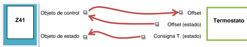
Figura 90 Consigna relativa (coma flotante). Enlazado de objetos.
