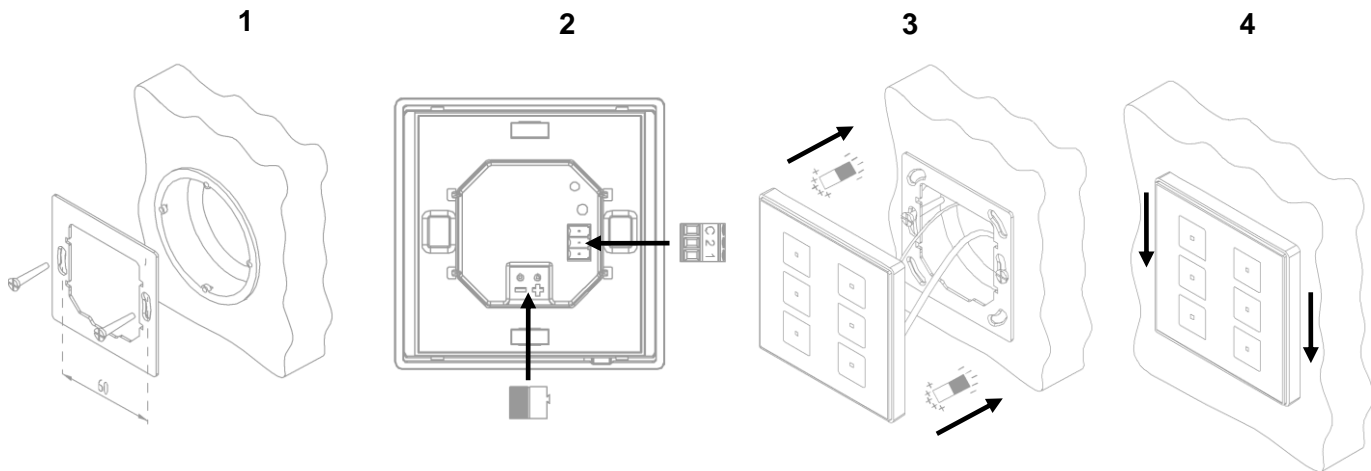
Figura 2 Instalación.
