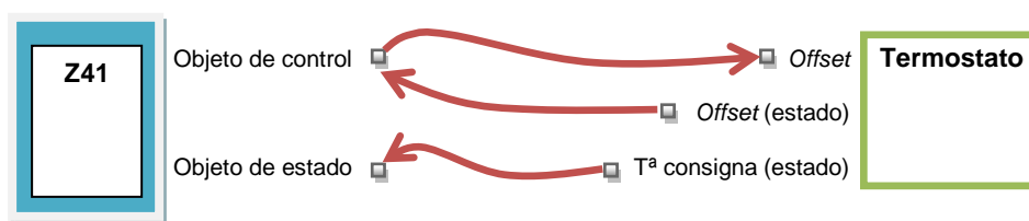
Figura 56 Consigna relativa (coma flotante). Enlazado de objetos.
