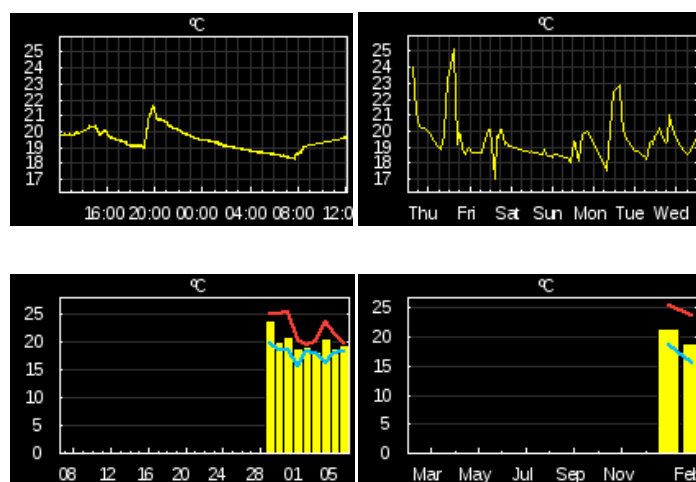
Figura 38 Diferentes niveles de detalle (log de datos)
