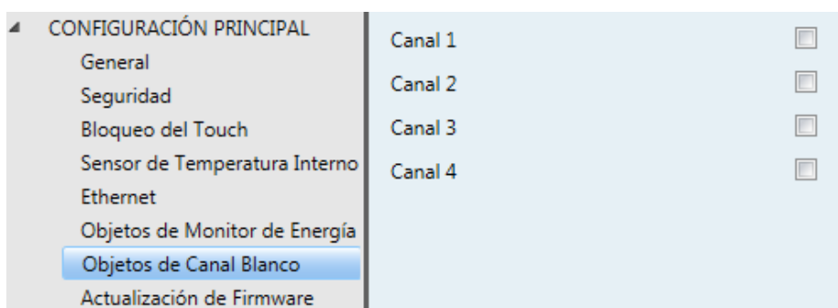
Figura 24 Objetos de canal blanco (Configuración principal)
