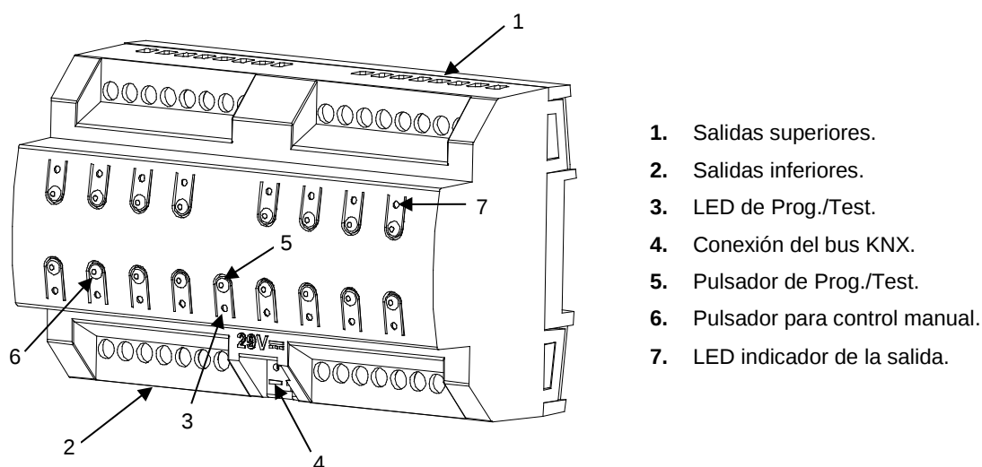
Figura 1. MAXinBOX SHUTTER 8CH. Elementos.
