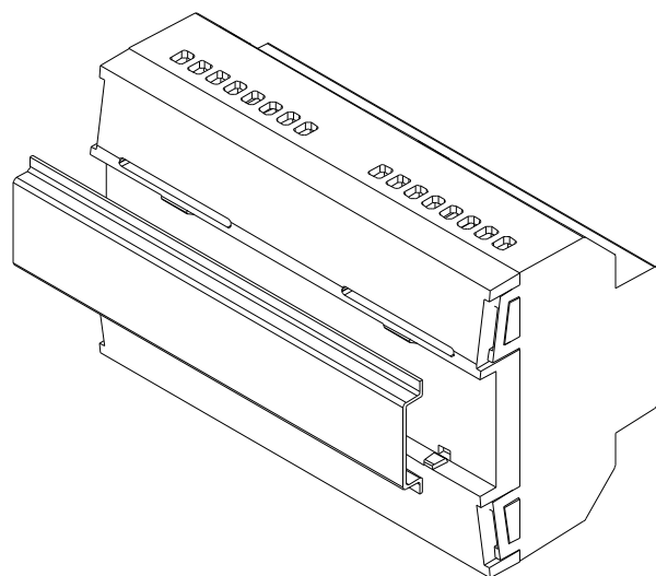
Figura 3. Montaje de MAXinBOX SHUTTER 8CH en carril DIN
