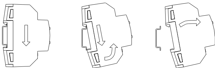
Figura 3. Montaje de MAXinBOX SHUTTER 8CH en carril DIN
