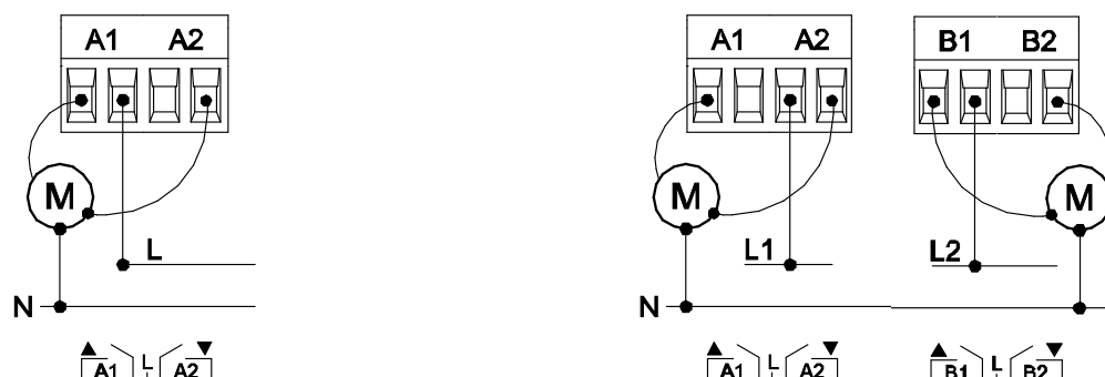
Figura 2. Ejemplo de conexionado (de izquierda a derecha): canal A y canal A y B con fases diferentes
