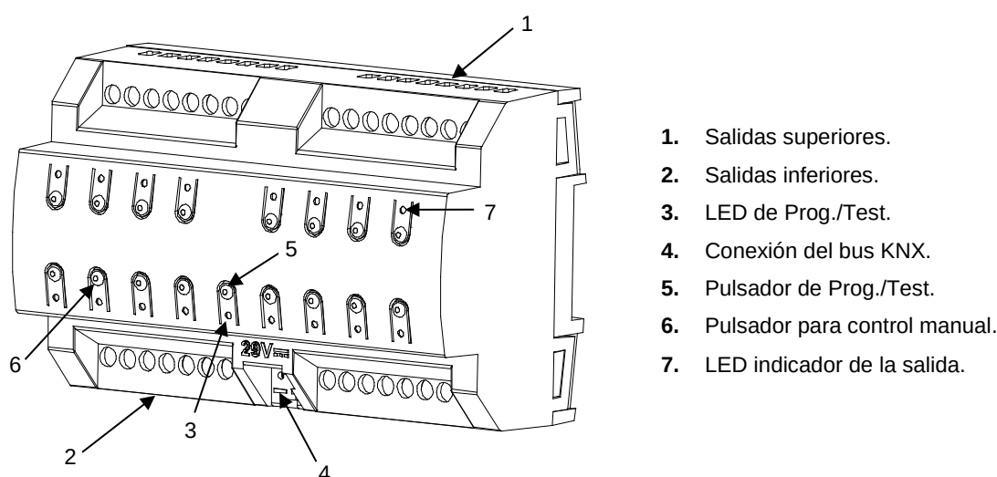
Figura 1. MAXinBOX SHUTTER 8CH. Elementos.
